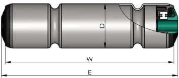
O带双槽输送辊筒
