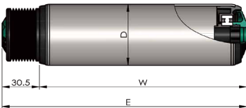
多楔带输送辊筒
